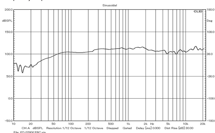
Frequency response curve in Enclosure (* 車両装着時のデータではありません。)
