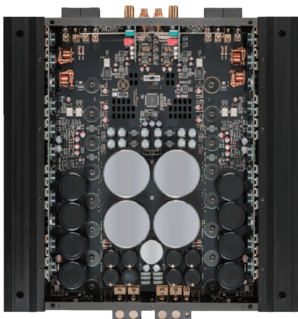
シンメトリレイアウト採用の内部基盤
